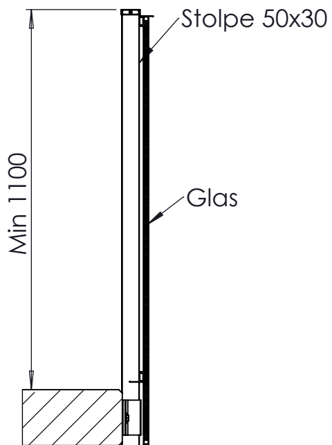
SECTION A-A SCALE 1 : 15
