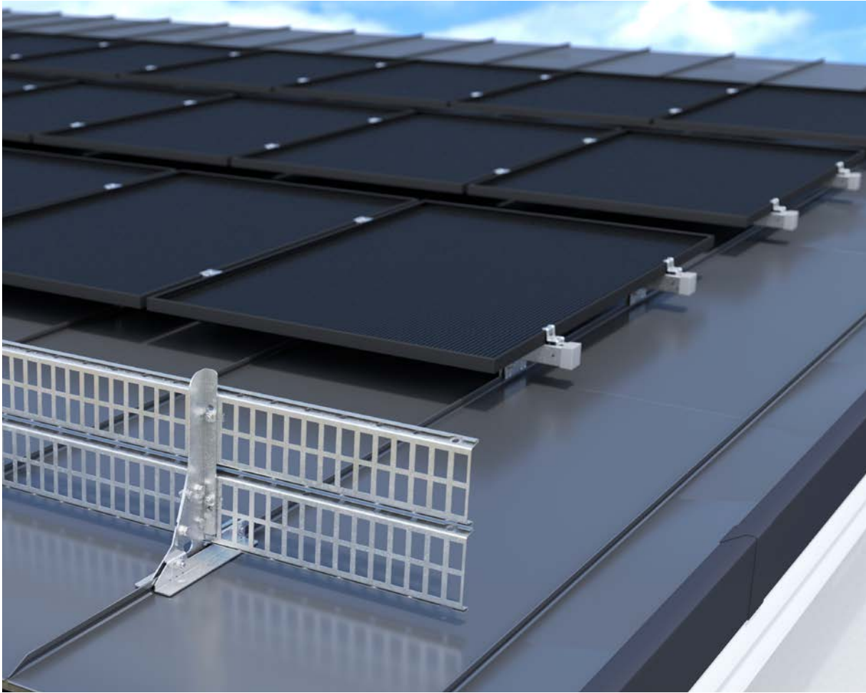
Forhøyningsfestefor snøfanger.
