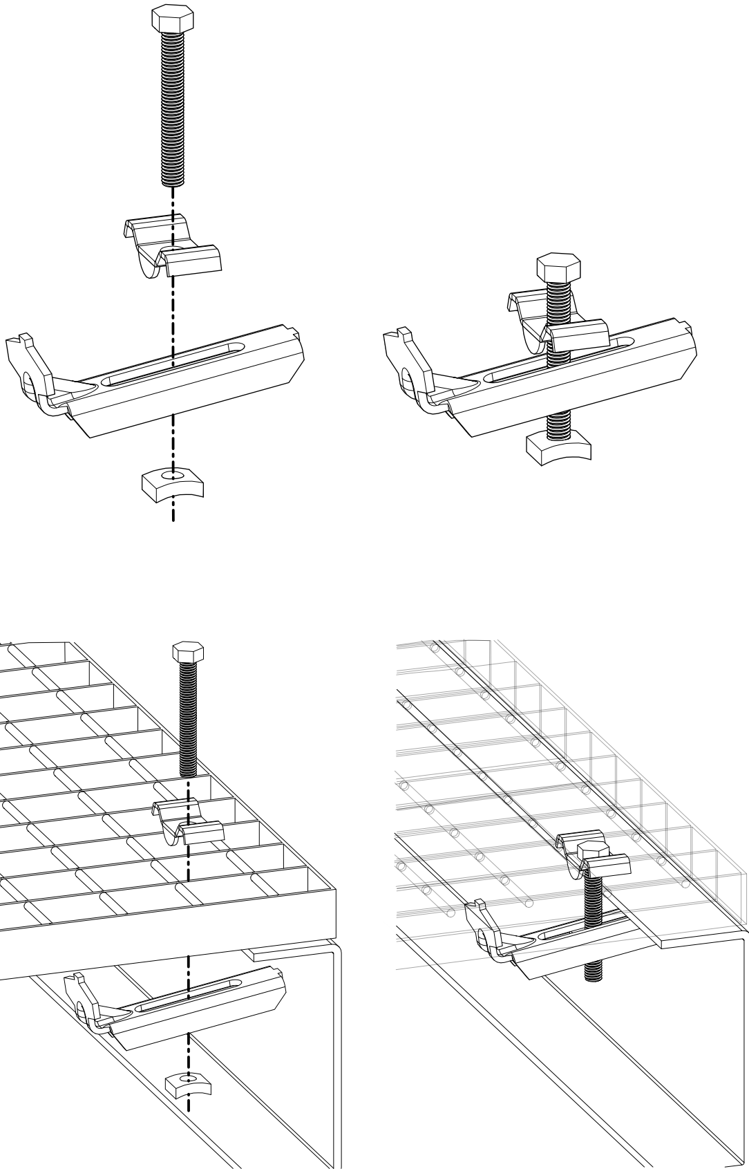
Montering av komplett festeklammer for gitterrist. Prinsipp viser H-rist og U-bjelke.
