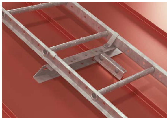
Falsfeste båndtekkning.
