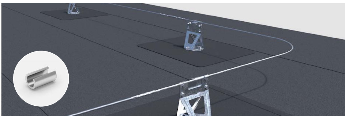
Vaierfeste til flate tak. Det innfelte bildet viser en klemhylse til hjørne (XWL 1014).
