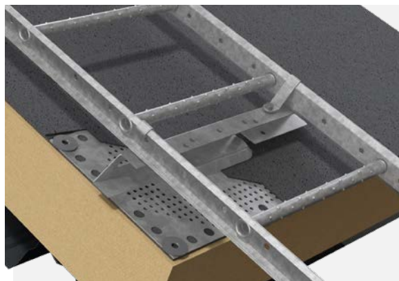
Festeplate for tettesjikt.
