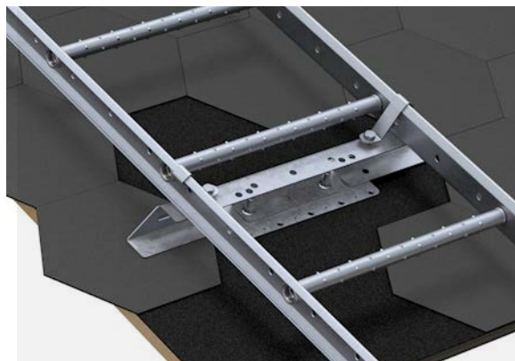
Festeplate på shingeltak.
