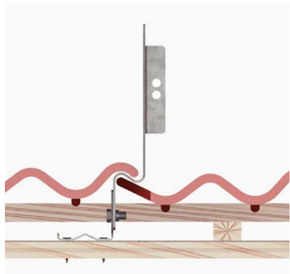
Tverrsnitt av holder for svensk teglstein.
