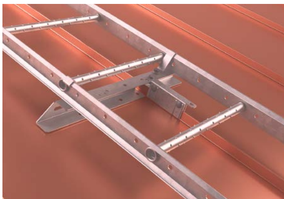
Falsfeste klikktak.
