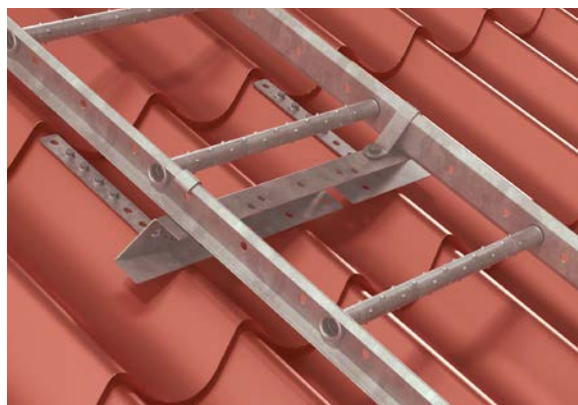
C-profil og innfestingsprofil for profilerte platetak.
