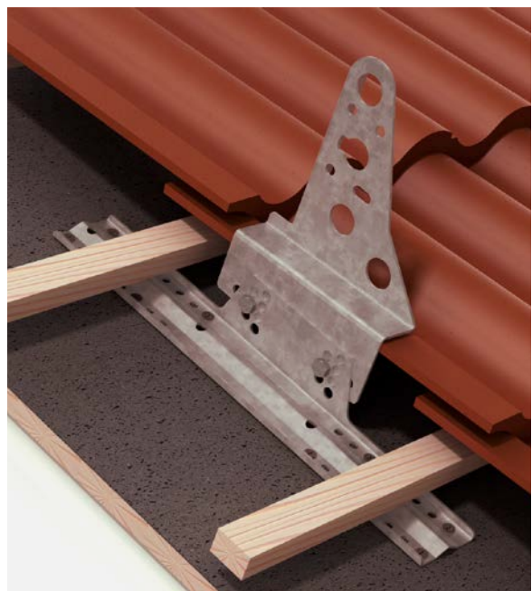
Innfesting med fotplate.
